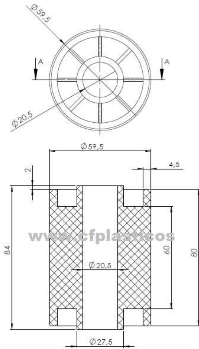
SEÇÃO A-A
